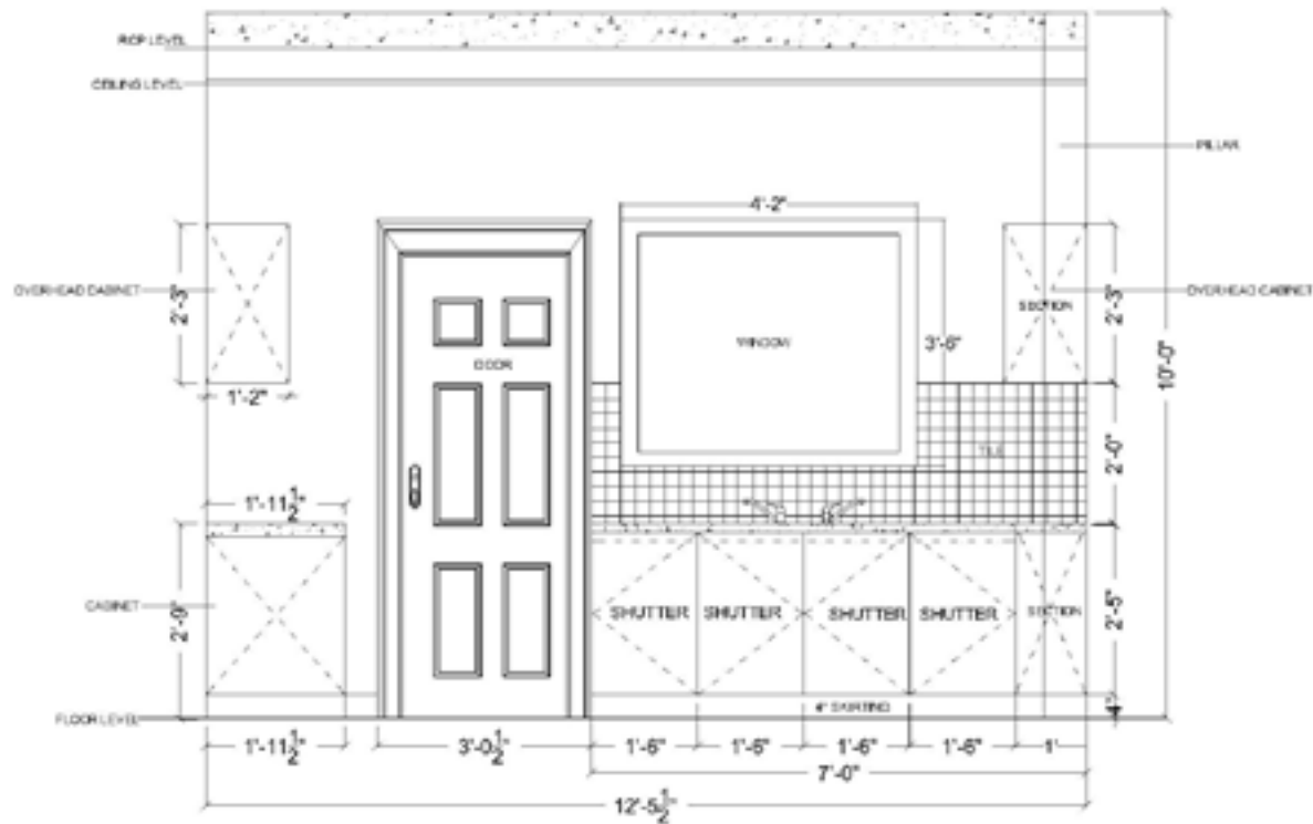
ELEVATION
